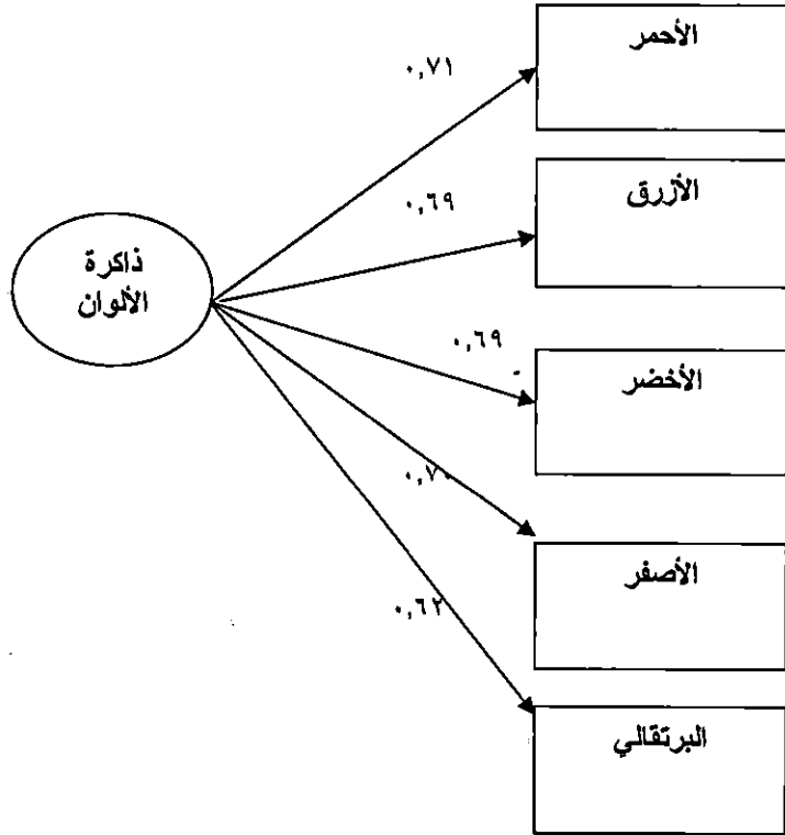
شكل (١) المسار التخطيطي لنموذج العوامل الكامنة لمقياس ذاكرة الألوان.
